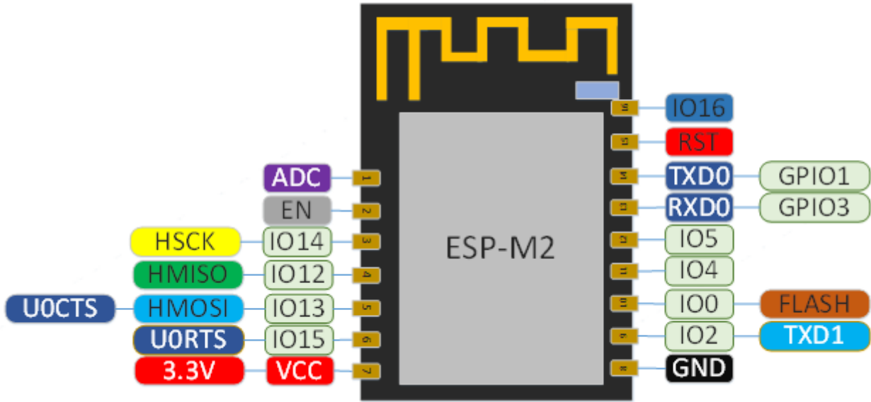
图 2.1 ESP-M2 Definition for Pins
